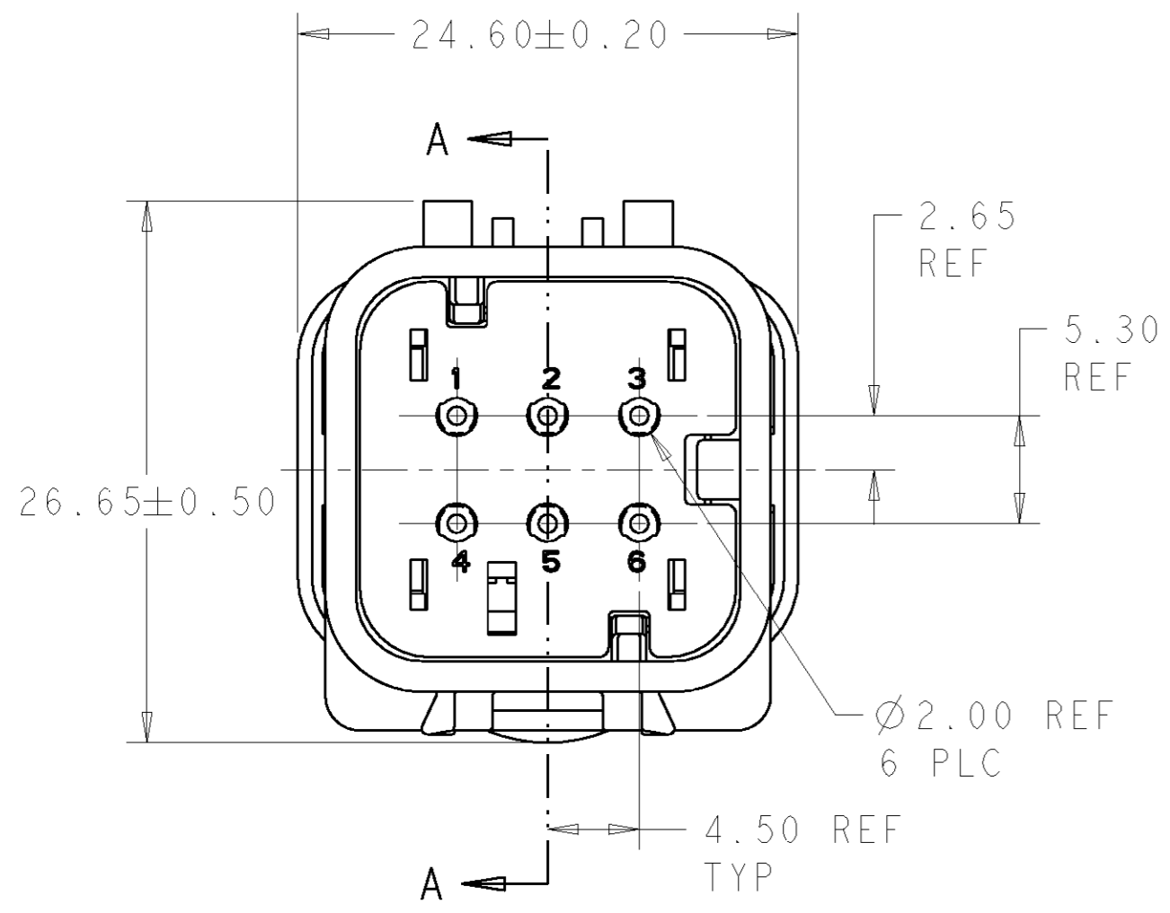
776537-1 SHOWN
