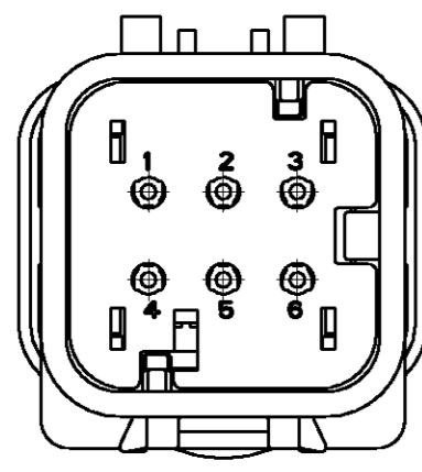
776537-2 SCALE 2:1
